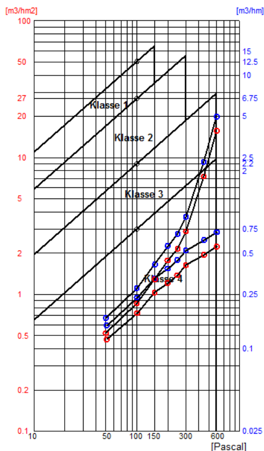
Figura 2 Diagrama de variatie a debitului de aer pierdut raportata la lungimea rosturilor si la suprafata esantionului
