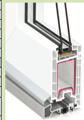
Sectiuni caracteristice
